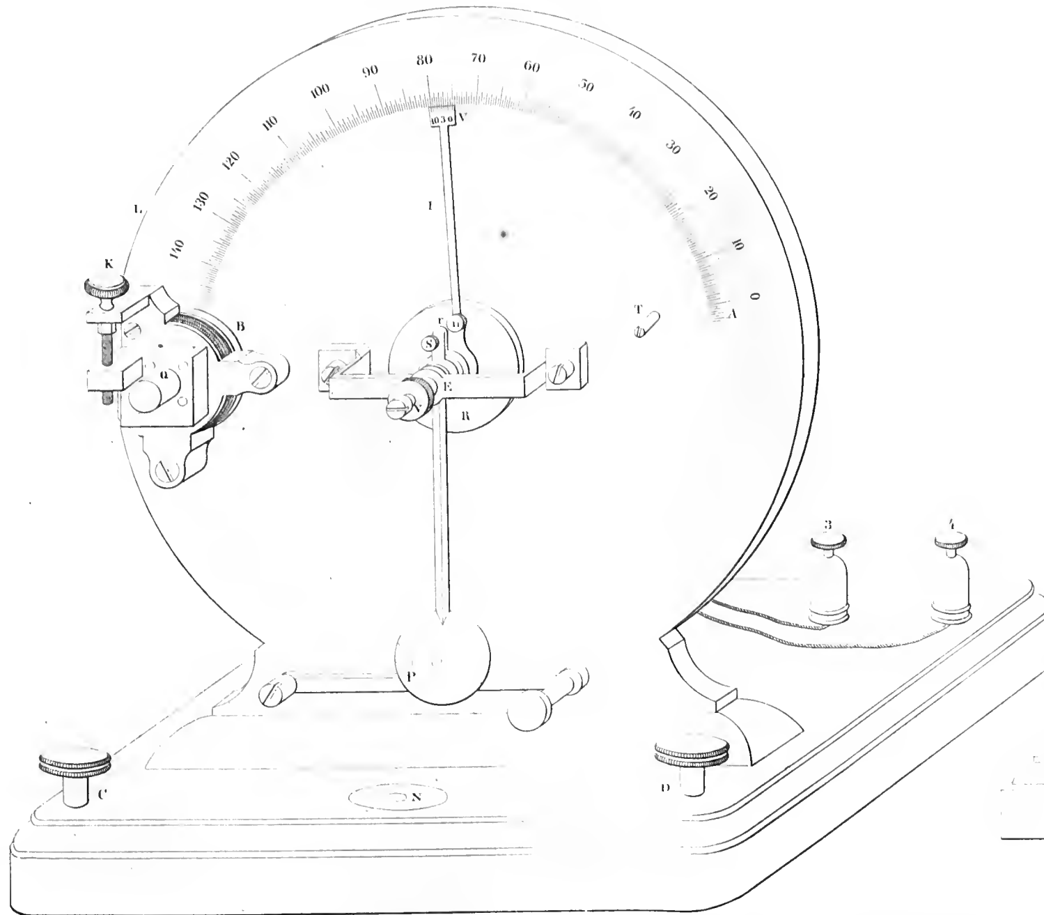
Pendulum
